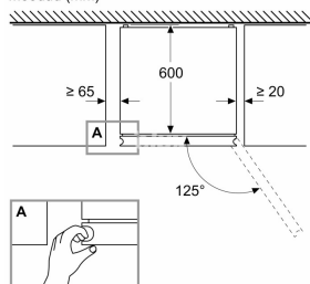
Mõõdud (mm)
