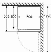
Mõõdud (mm)
