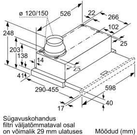
Mõõdud (mm)
