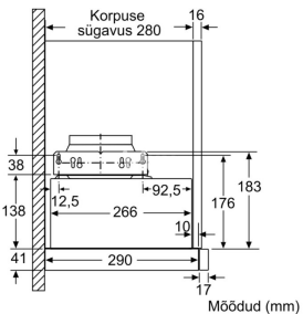
Mõõdud (mm)
