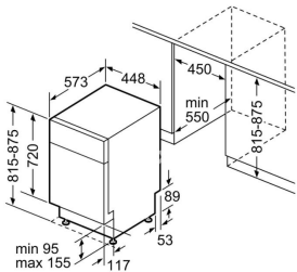
mõõdud (mm)
